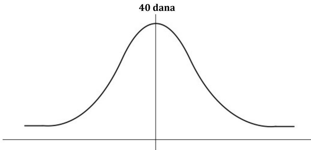
Slika 1. Normalna raspodela
